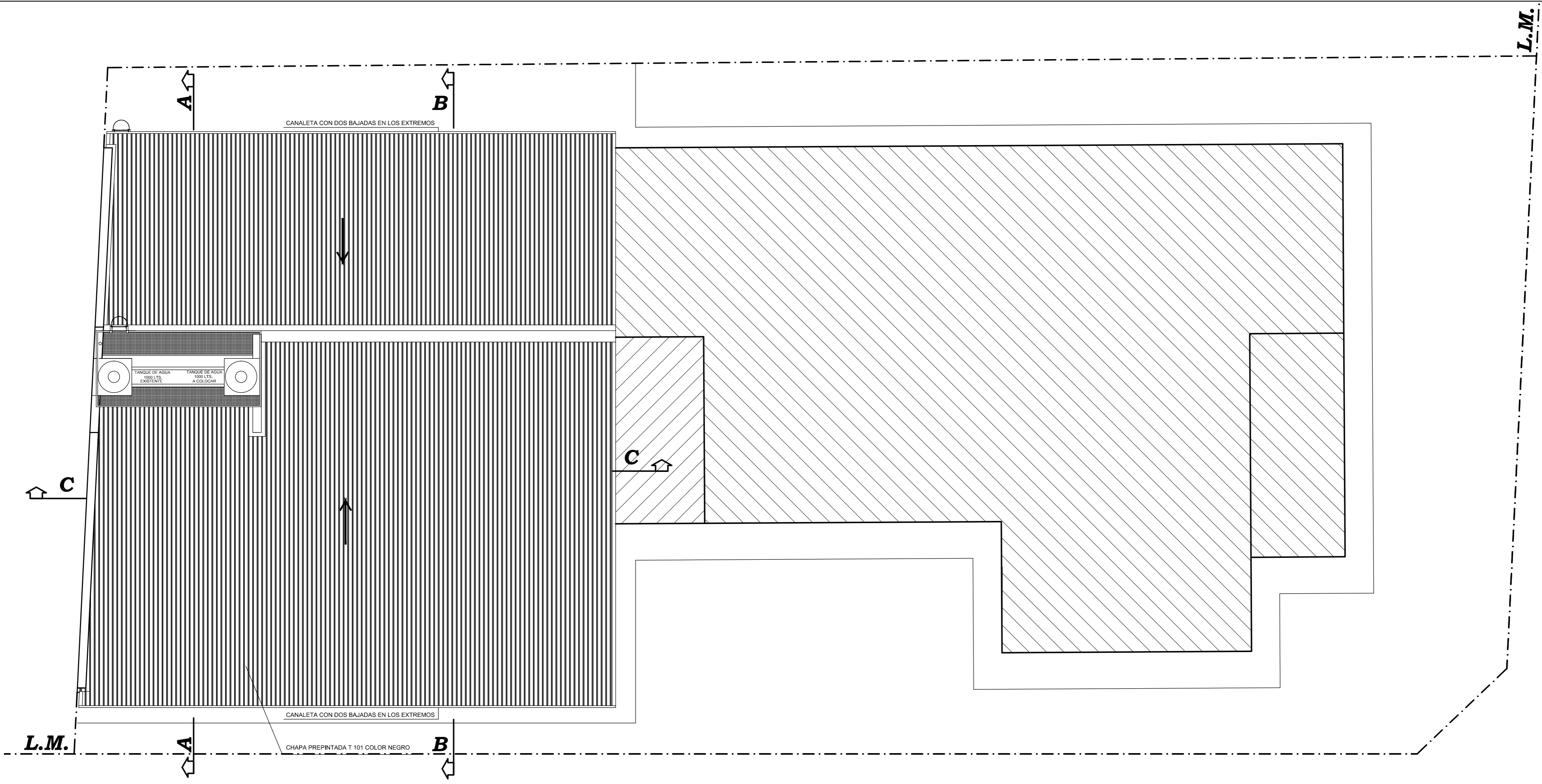
PLANTA TECHOS
